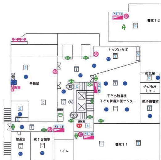
1 階
