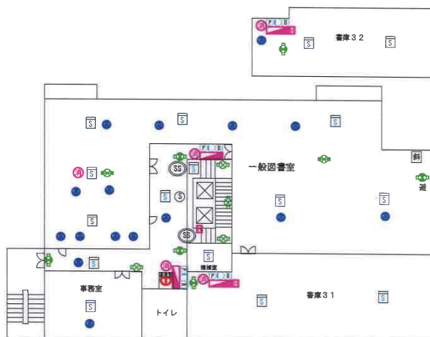
3 階
