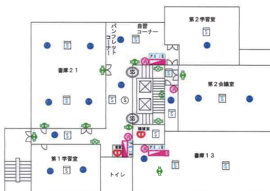
2 階
